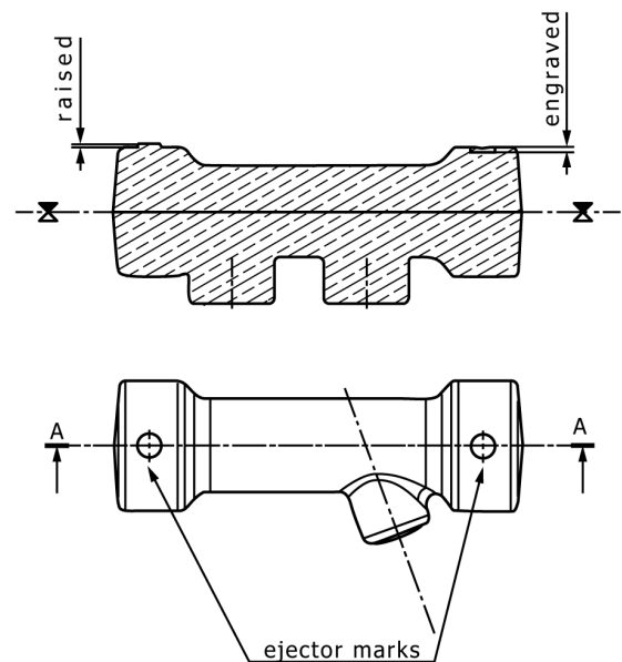
FIG. X2.3 Ejector Marks
